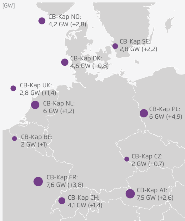
Cross-Border-Kapazität (CB-Kap)
